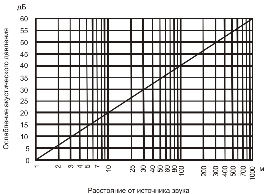
Рисунок 12.1 — График зависимости ослабления звукового давления от расстояния до источника звука».
